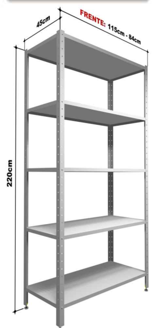
ESTANTE ABIERTO
