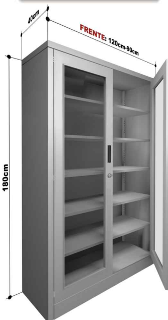
2 PUERTAS ENMARCADAS
